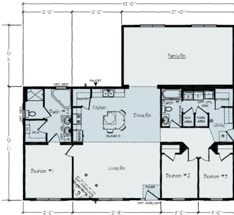
Optional Floor Plan B
